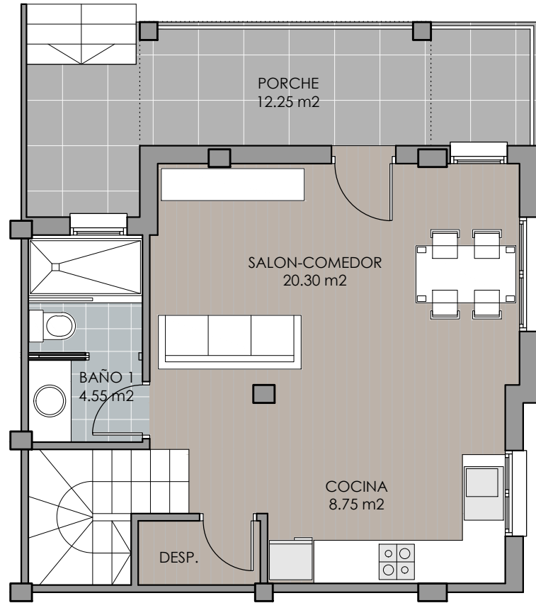
PLANTA BAJA 1:75
