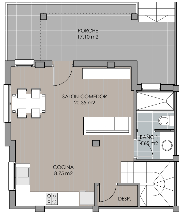
PLANTA BAJA 1:75
