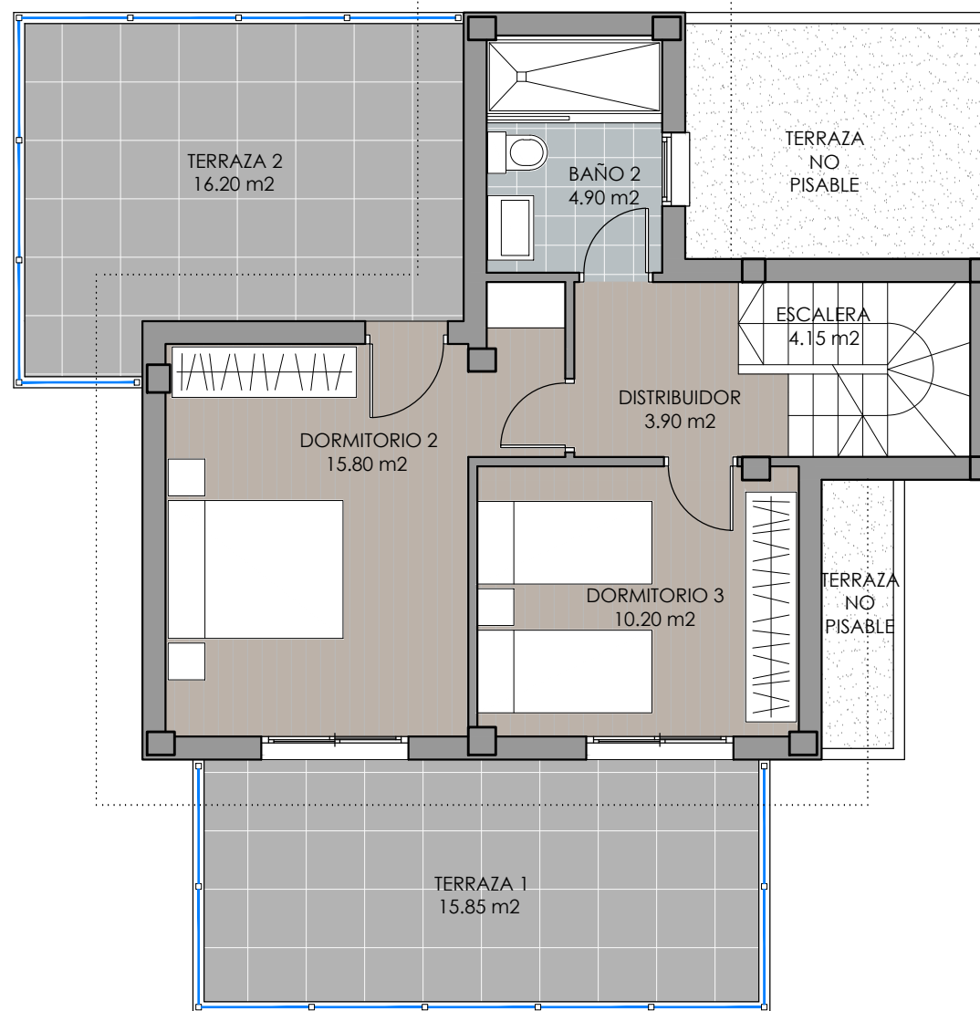
PLANTA ALTA 1:75
