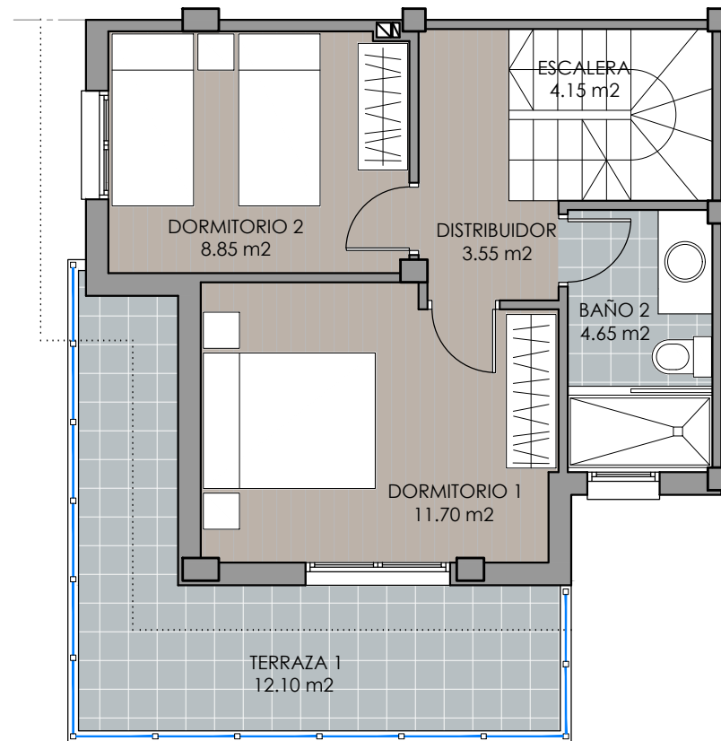
PLANTA ALTA 1:75
