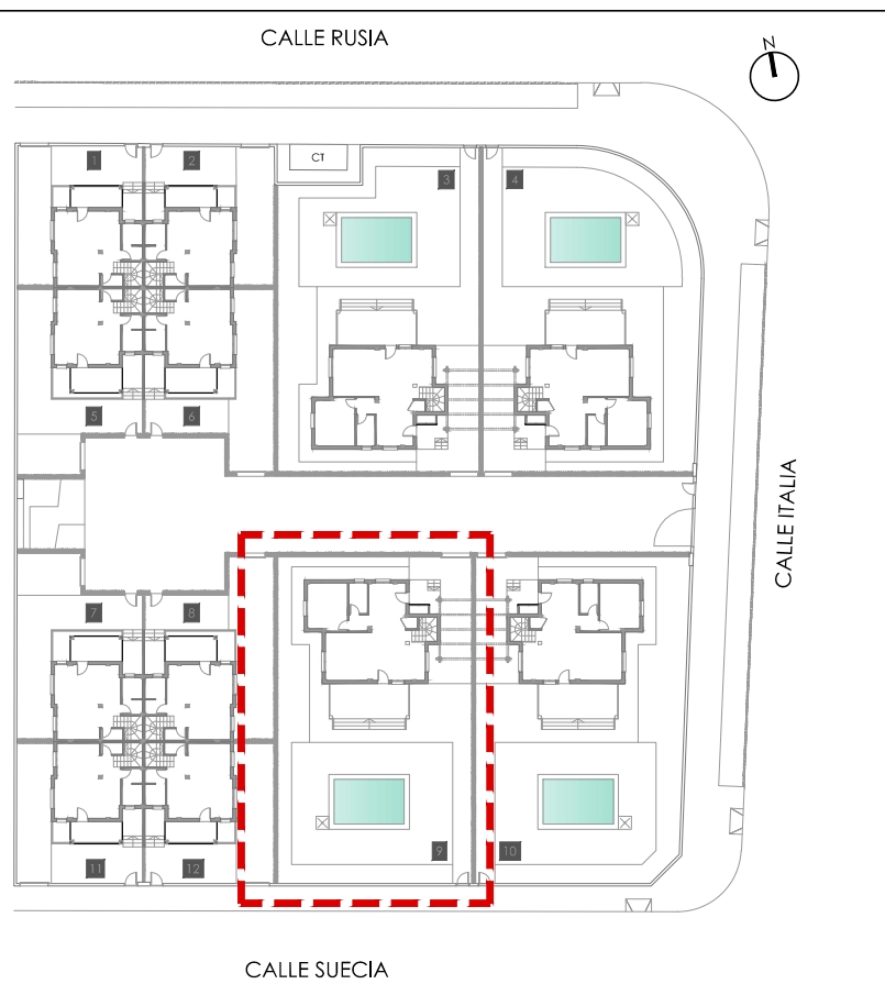
PLANTA BAJA 1:75
