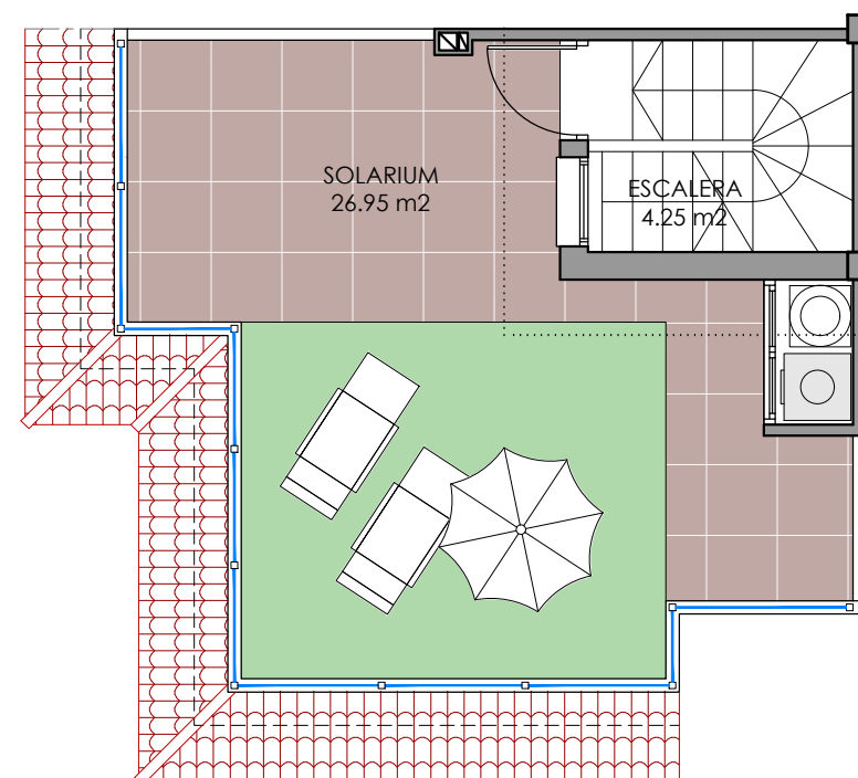
SOLARIUM 1:75
