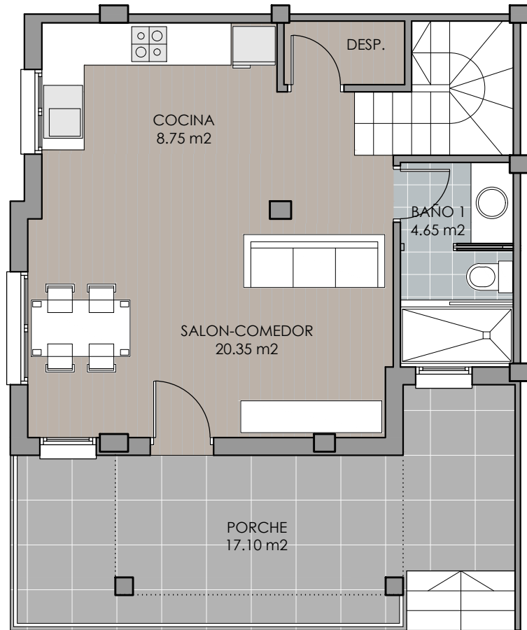
PLANTA BAJA 1:75
