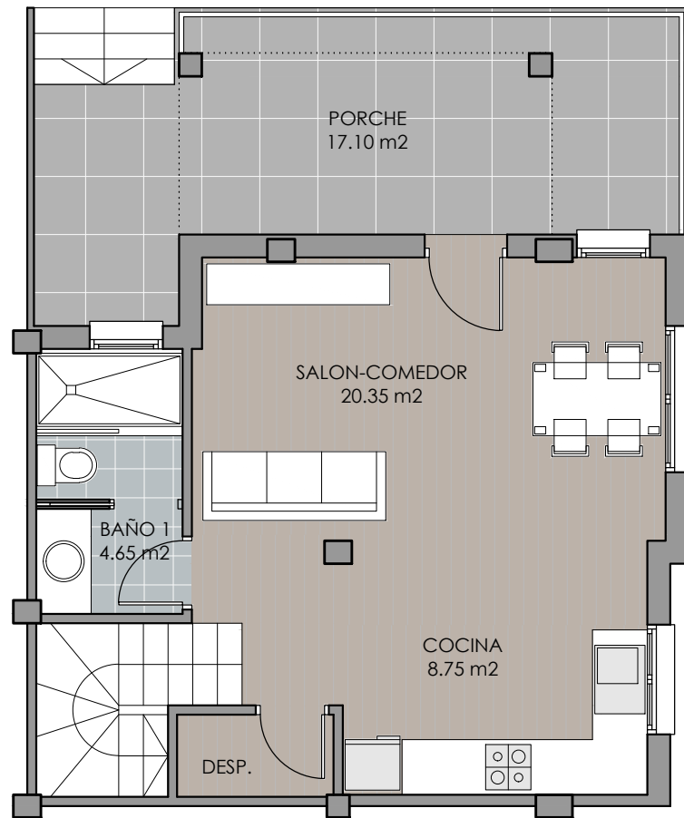
PLANTA BAJA 1:75
