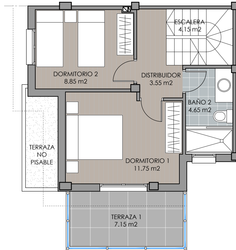
PLANTA ALTA 1:75
